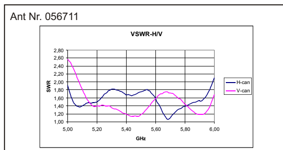
VSWR
